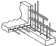
Juntas de construcción en concreto
